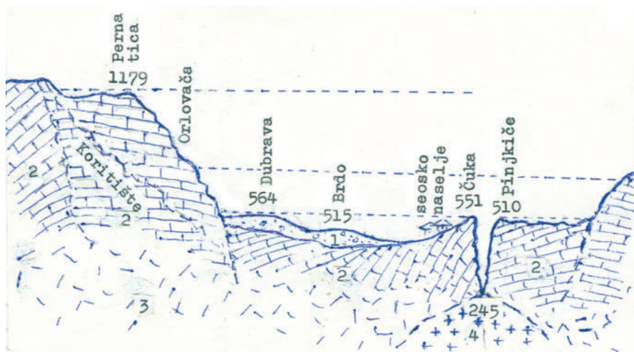
Попречни профил источног дела Сићевачке клисури на линији Пернатица (1179 m) – Пикњице (510 m). Главни абразиони и доњи језерски под (језерско дно) приказани су цртицама:
